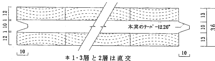
図1 断面形状図
